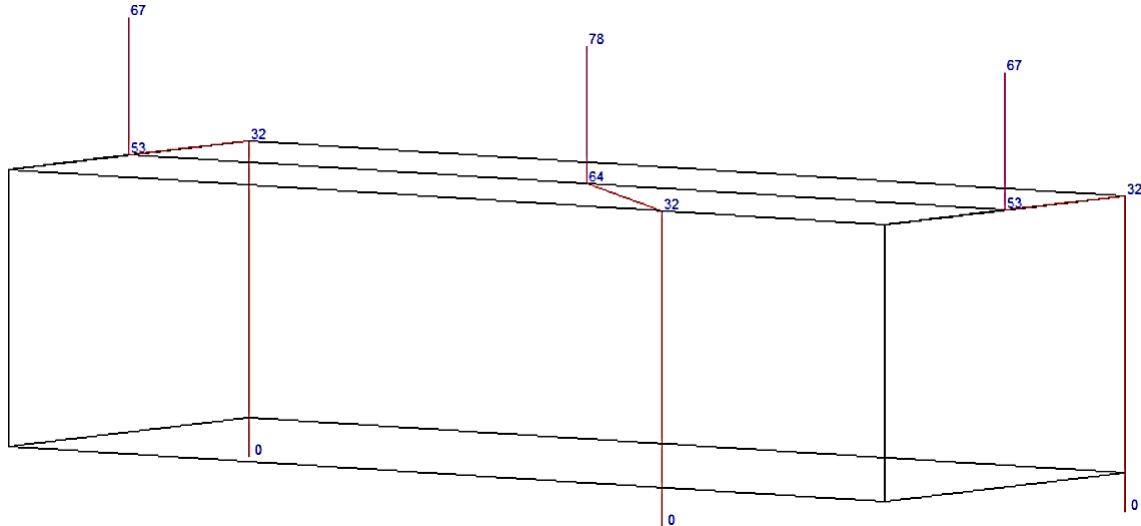
Zjednodušená simulace dostatečné vzdálenosti „s“ (v cm) pro vrcholový proud 100 kA (LPS III) dle ČSN EN 62305-3 ed. 2 pro k_m = 1 (izolace vzduchem); pohled na objekt od jihu (v simulaci není modelována šikmá střecha, ale pouze skutečná trasa navržených izolovaných vodičů)
