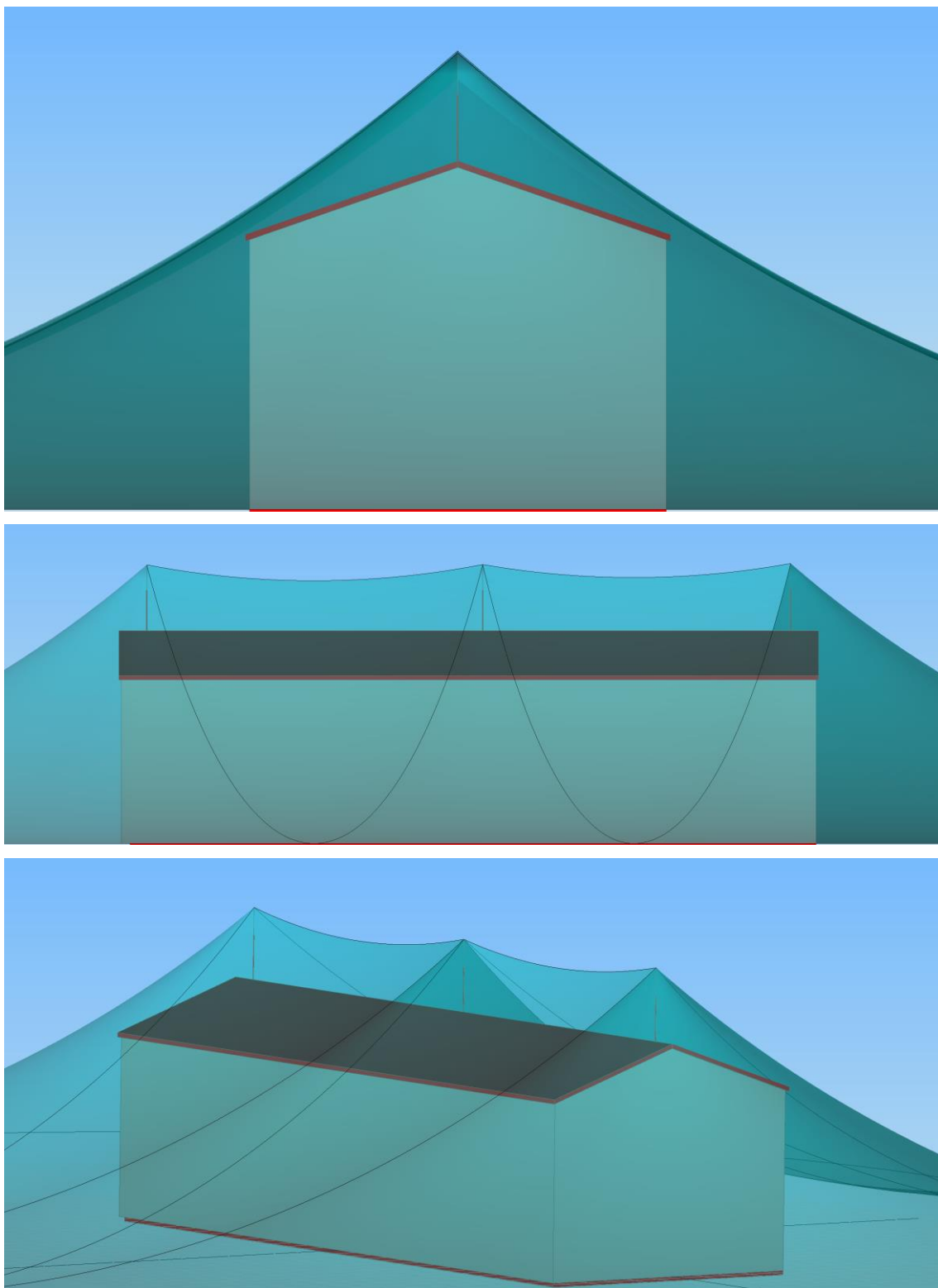
Ověření návrhu pomocí simulace ochranných prostor valivými koulemi dle ČSN EN 62305-3 ed. 2 pro LPS III
